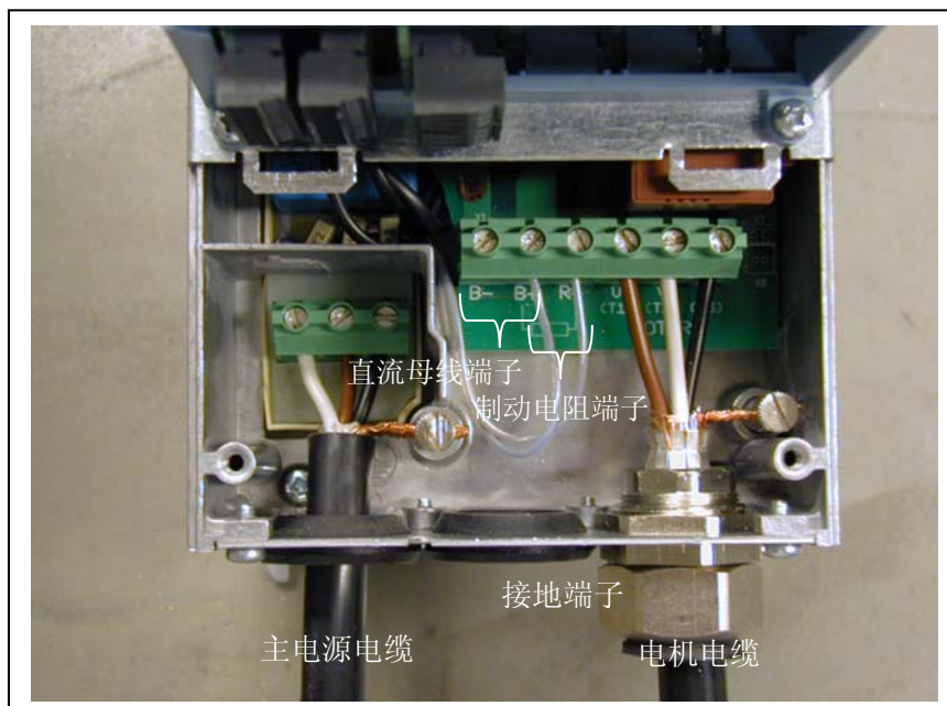
图 6-16. Vacon NXL 的电缆连接, MF4
