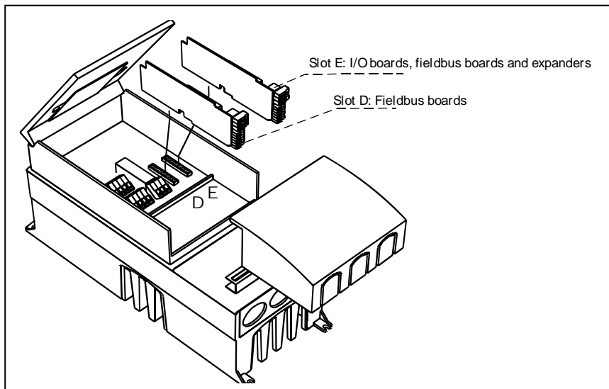
图 6-21. MF4–MF6 变频器的选件卡插槽 D 和 E
