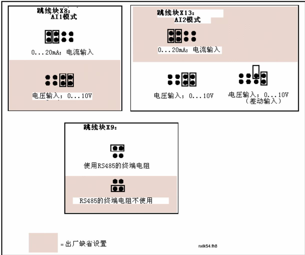
图 6-25. Vacon NXL 变频器的跳线选择, MF4-MF6
