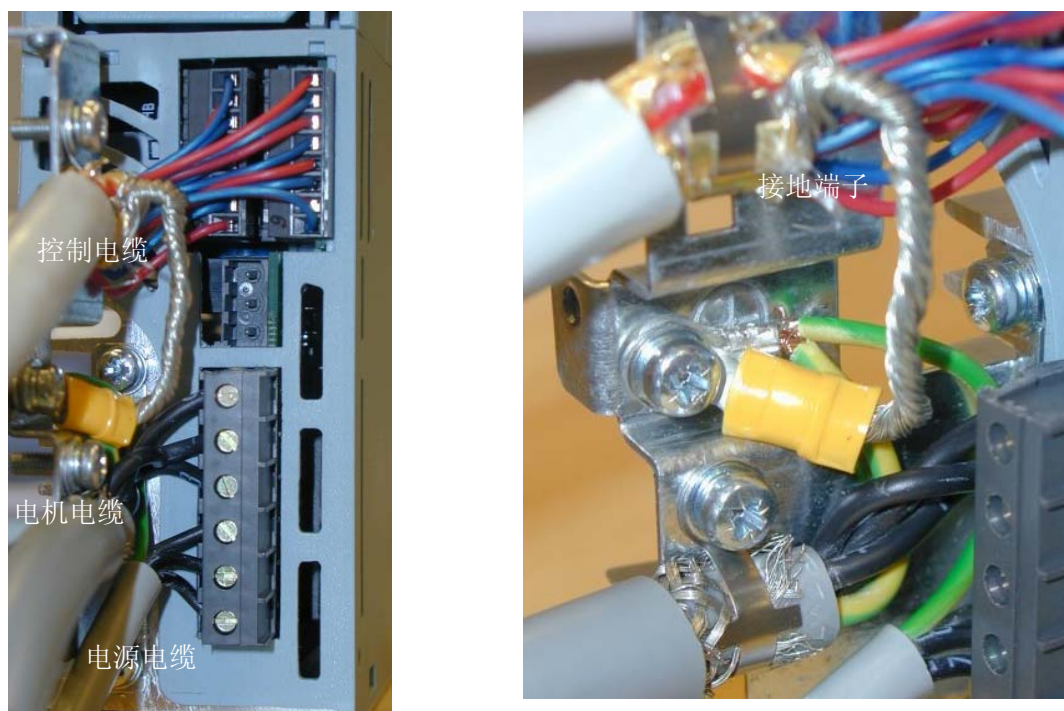
图 6-7. MF2 变频器的电缆安装 (500V, 3~)
