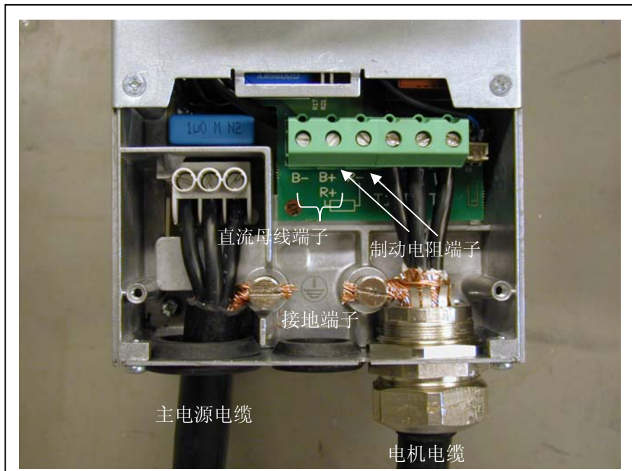
图 6-18. Vacon NXL 的电缆连接, MF5
