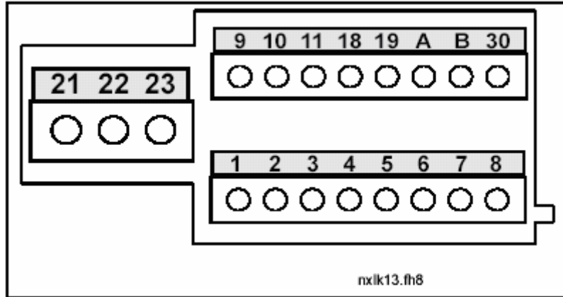
图 6-22. 控制信号连接, MF2-MF3
