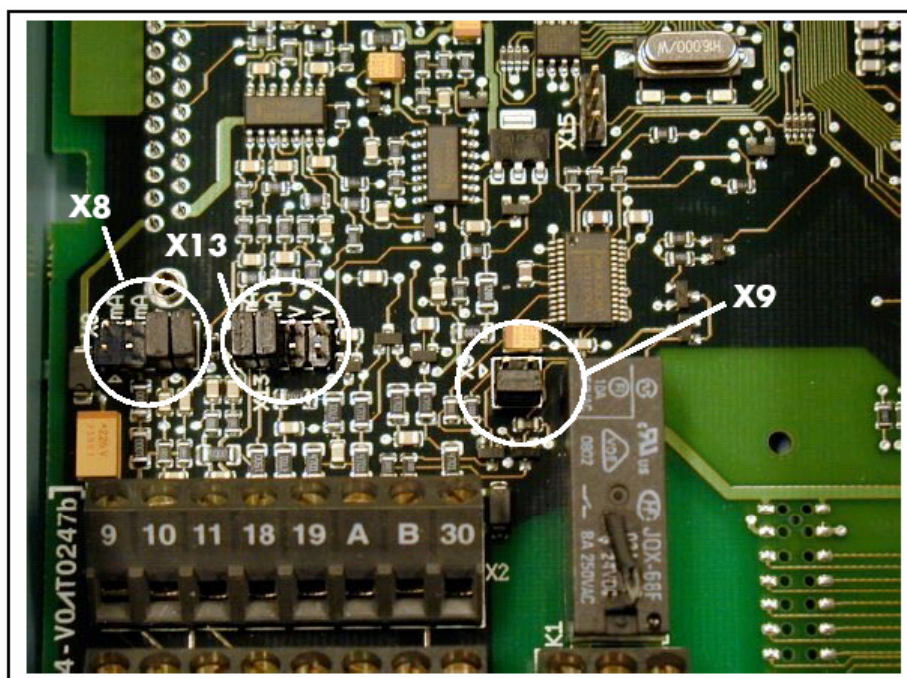
图 6-27. MF4—MF6 变频器控制板上的跳线位置
