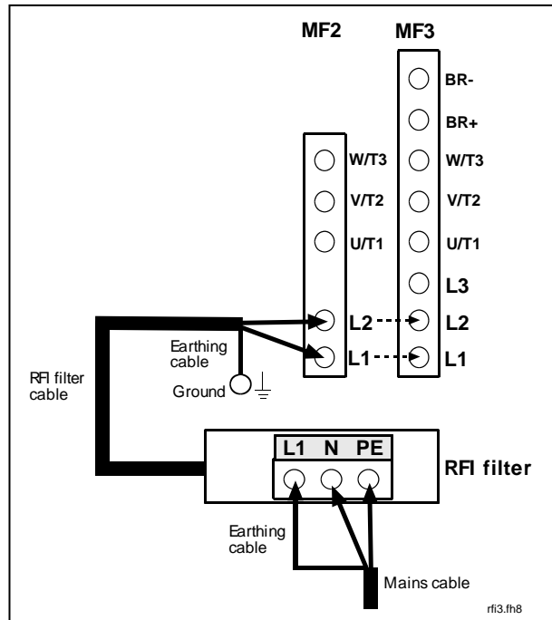
图 6-14. MF2 和 MF3 变频器的 RFI 滤波器电缆安装 (208...240V, 单相供电, 滤波器型号 RFI-0012-2-1)
