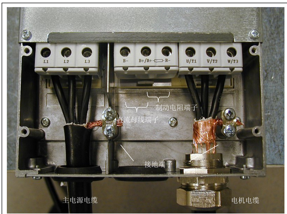
图 6-20. Vacon NXE 的电缆连接, MF6
