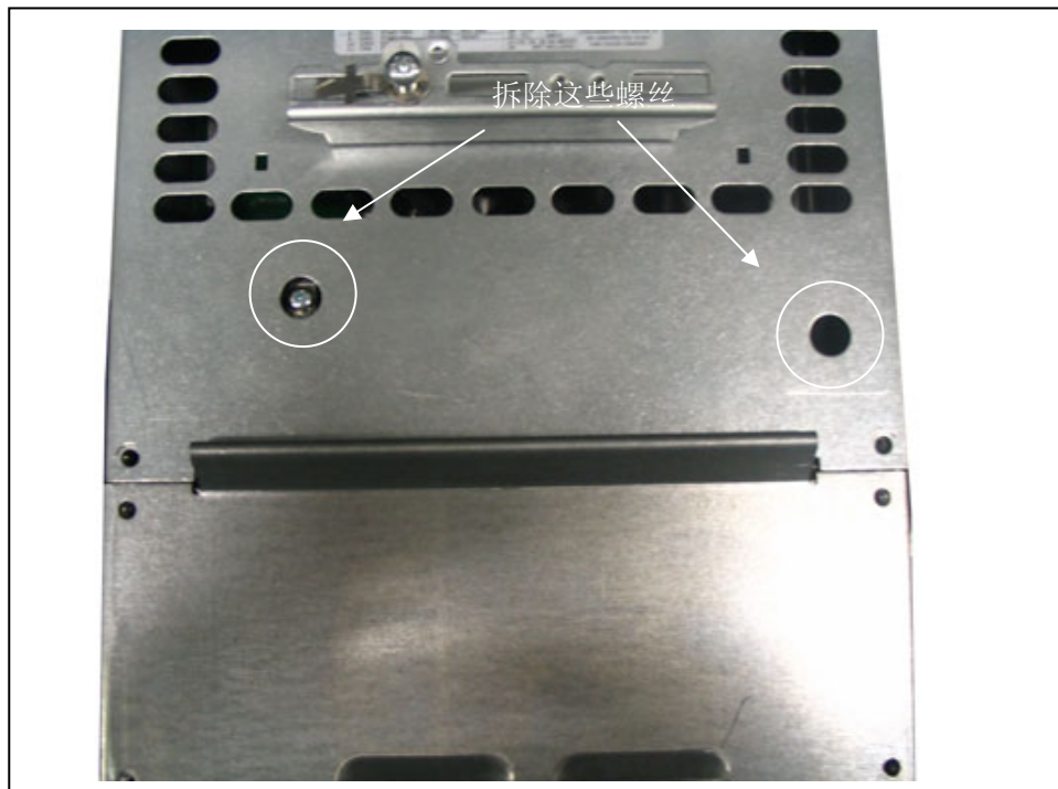
图 5-8. 改变 EMC 防护等级，MF6
