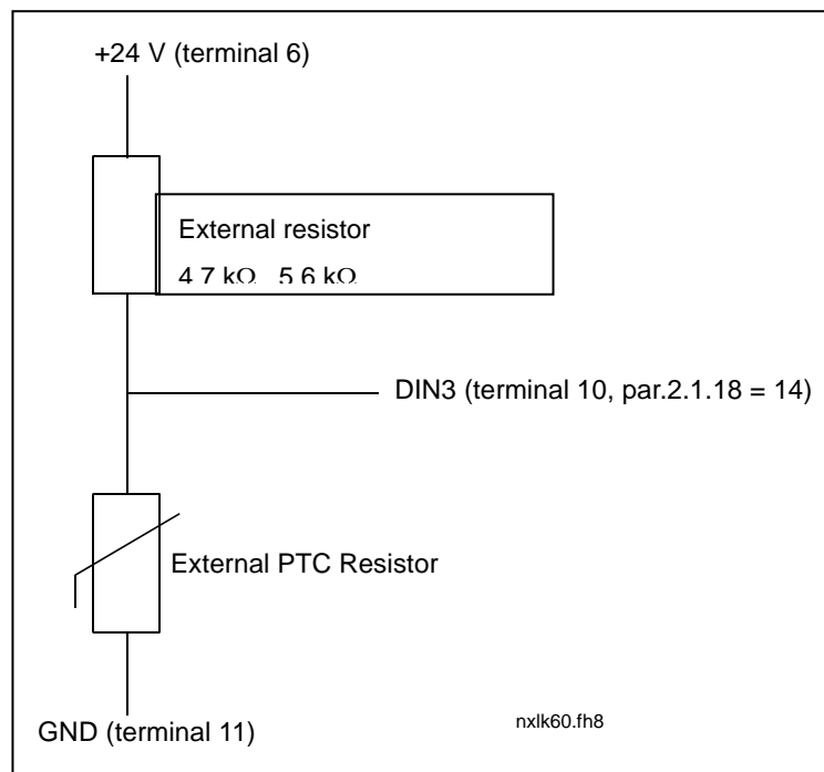
图 6-28. 电机热敏电阻 (PTC) 的连接
