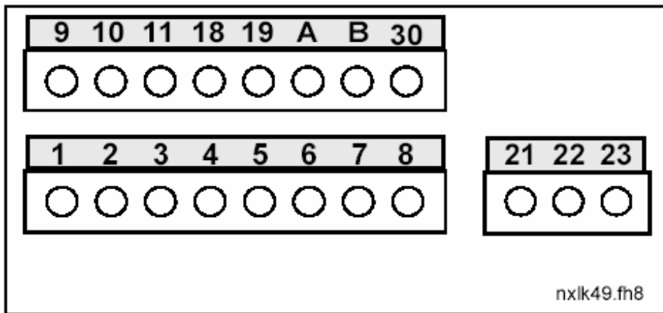
图 6-23. 控制信号连接, MF4-MF6
