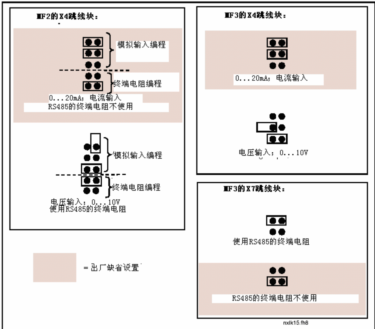
图 6-24. Vacon NXL 变频器的跳线选择, MF2 和 MF3
